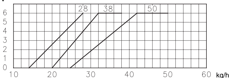
(F) Heizöldurchsatz in 2° Stufe / Light oil delivery in 2nd stage Débit fioul à la 2e allure / Oliedebiet in 2de vlamgang
