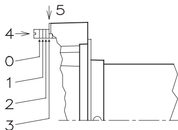
(F) ↓ N° Kerben - Notches - Encoches - Inkepingen
